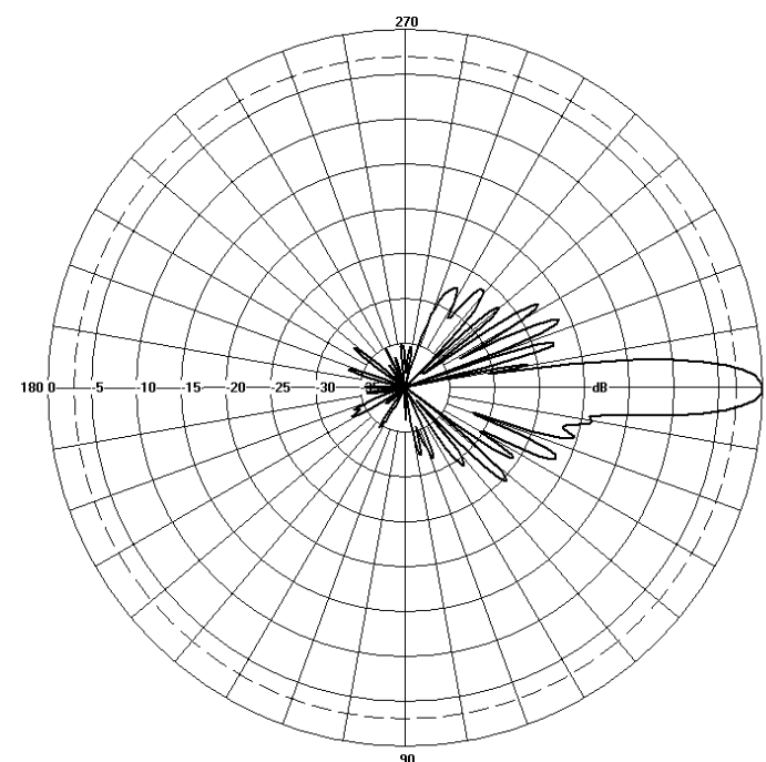
Elevation
