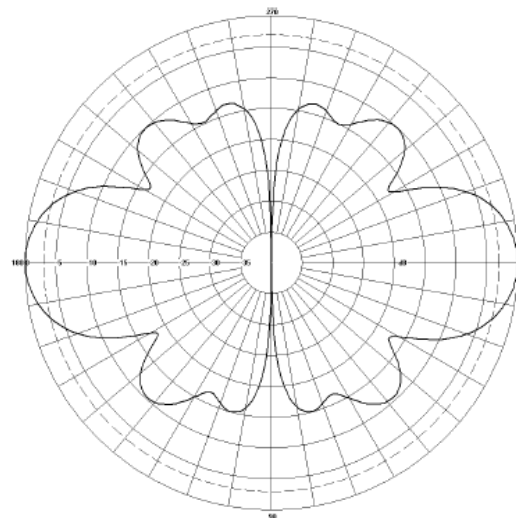
1710 - 2690MHz
