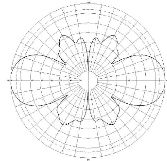
3400 - 3800MHz
