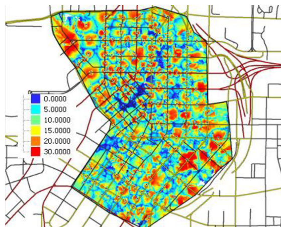
Fig. 10 – VT External Antenna SINR (dB)
